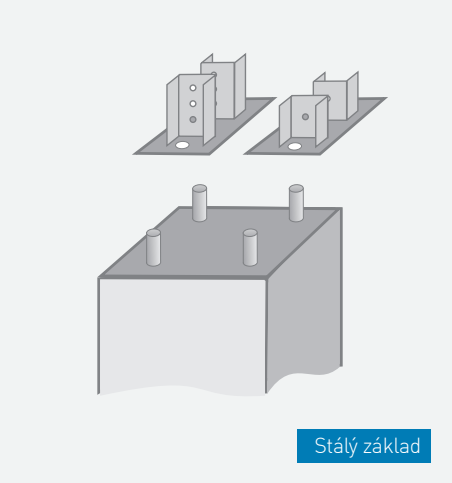
Prefabrikovaný základ
